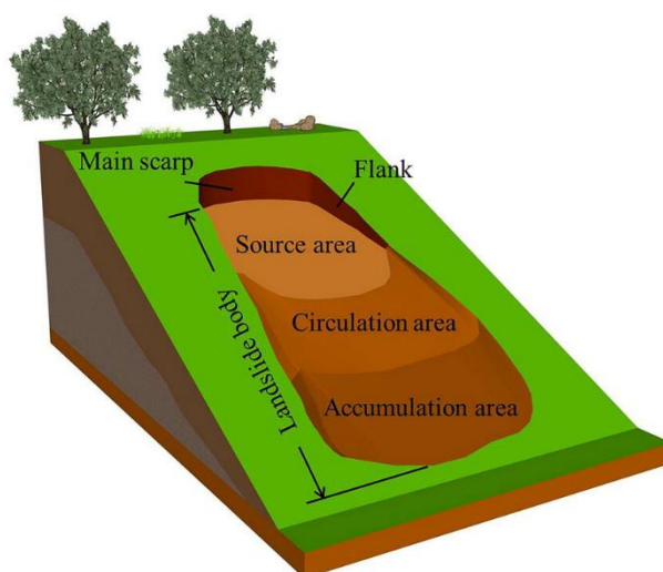
รูปที่ 2.3 กลไกและพฤติกรรมเคลื่อนไถของหน้าดิน
